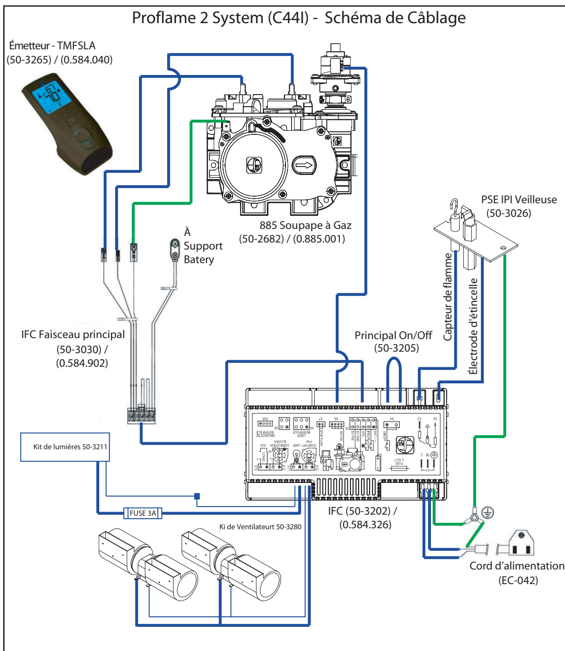
Figure 51: Schéma de Câbles du C60I
