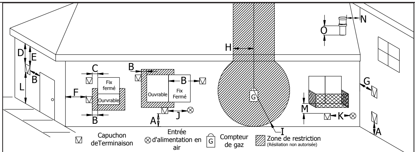
Figure 39. Résiliation d'événement des restrictions, reportez-vous à Tableau 3
