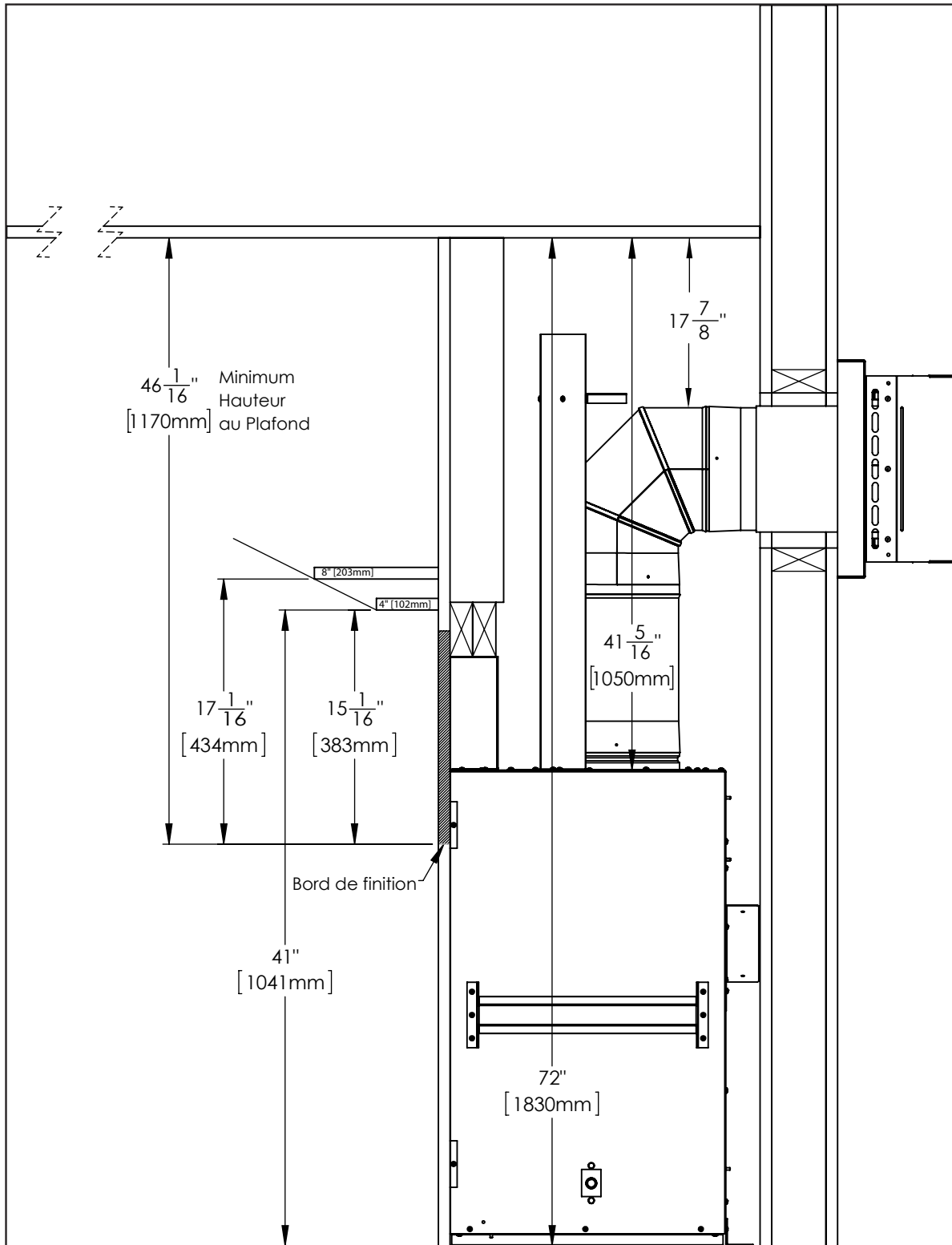
Figure 30(b): Dimension d'Installation avec Manteau
