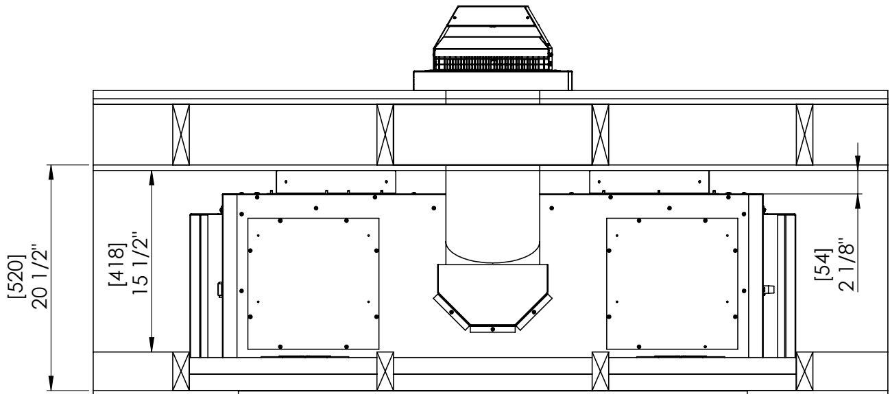
Figure 34(a). Dimensions d'un installation horizontal
