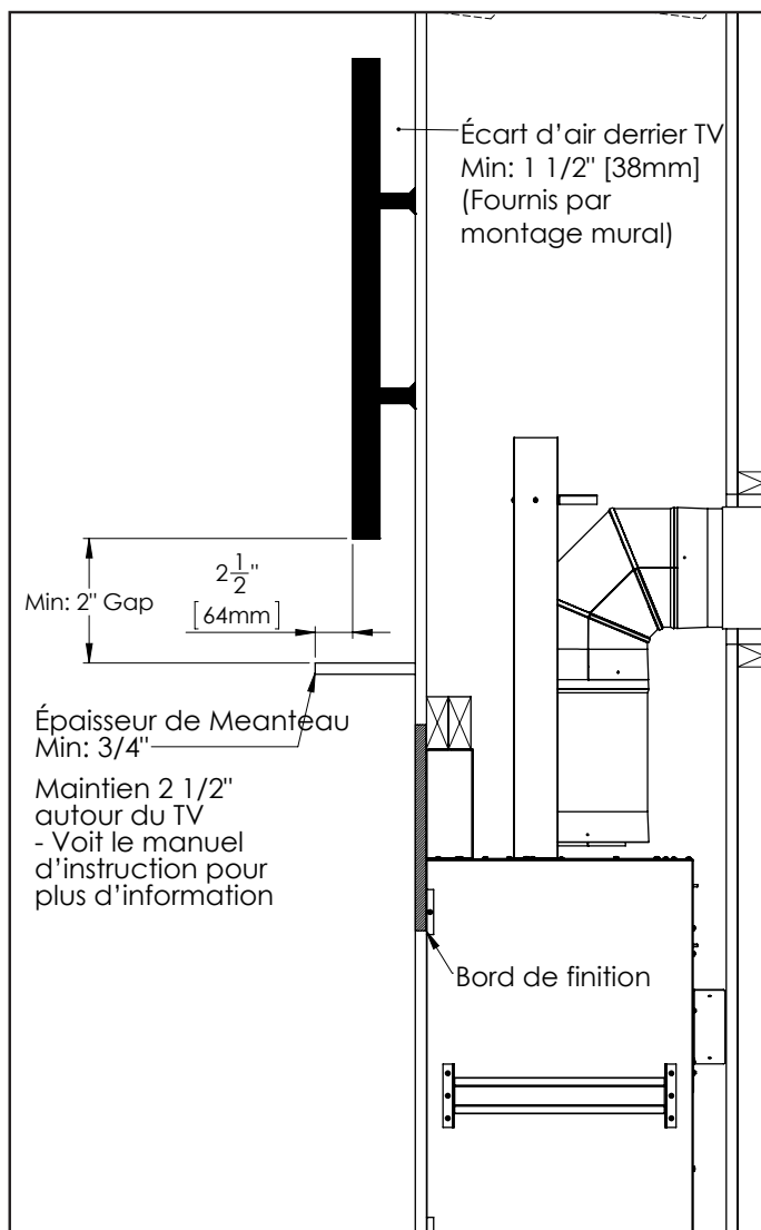
Figure 37. Dégagement Minimum d'Installation de TV
