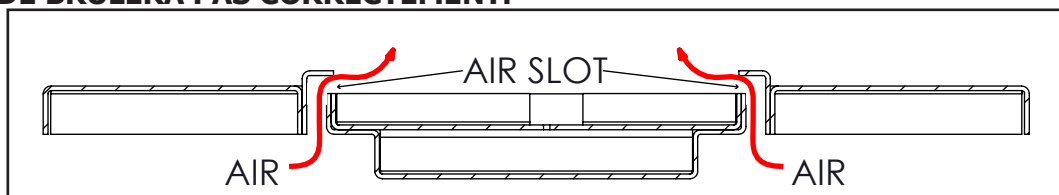
Figure 60 : Coupe transversale côté brûleur
