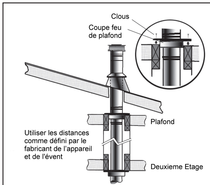
Figure 49: Installation des conduits à plusieurs étages
