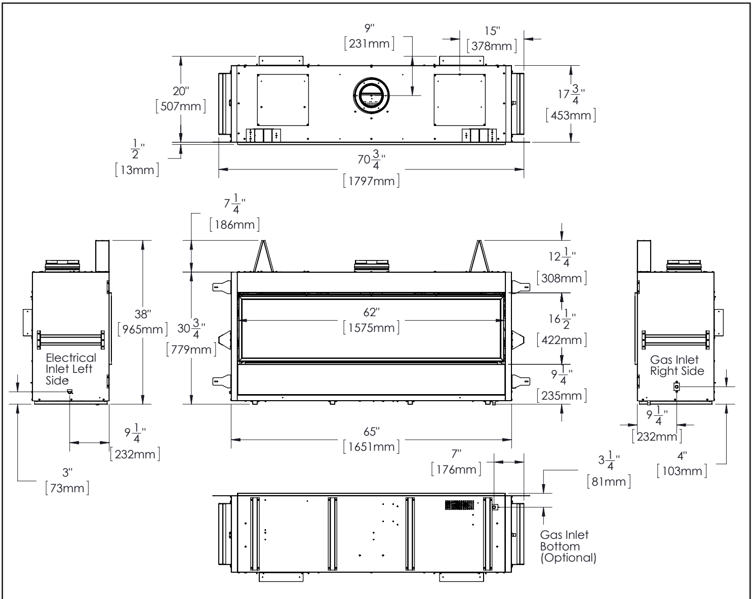
Figure 1. Dimensions du C60I
