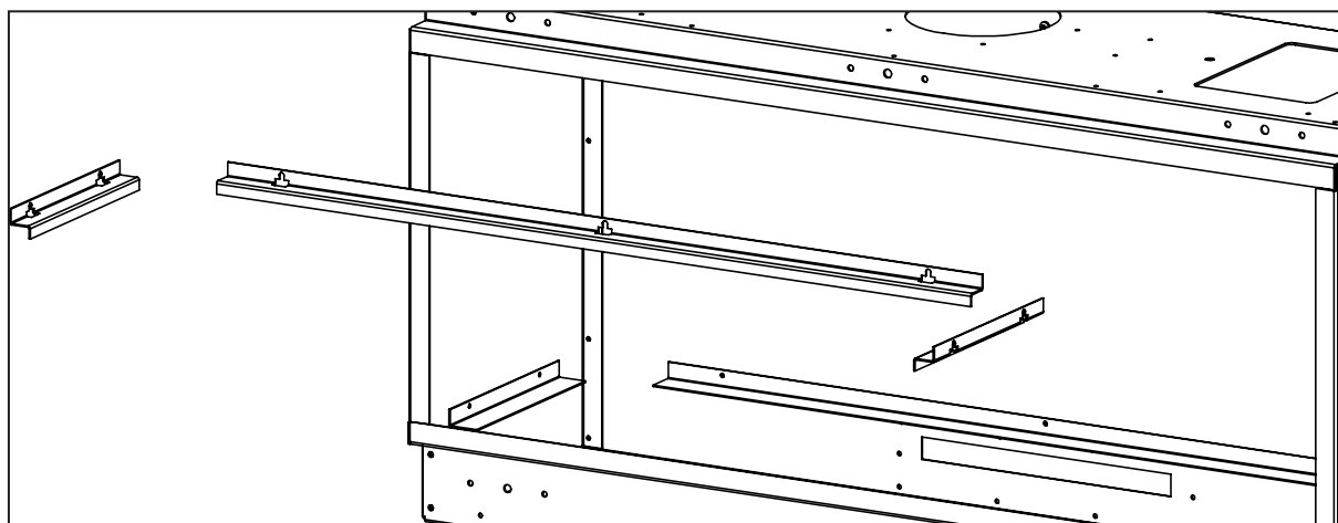
Figure 57: L'installation du panneau
