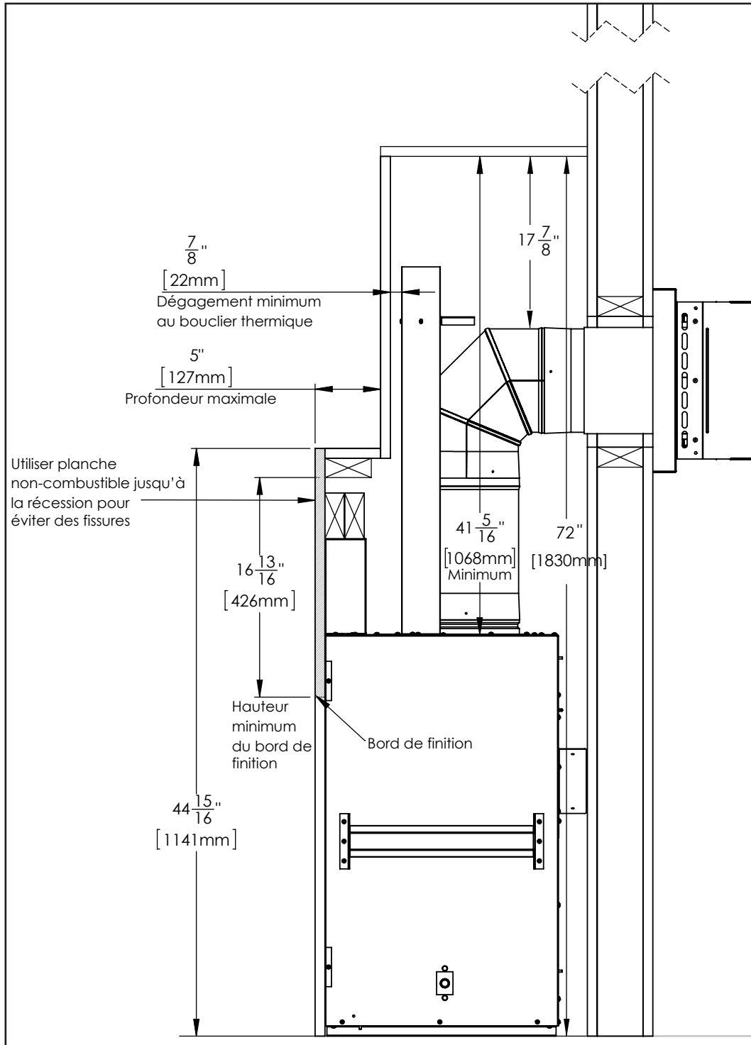
Figure 31: Dimension d'Installation du Renforcement
