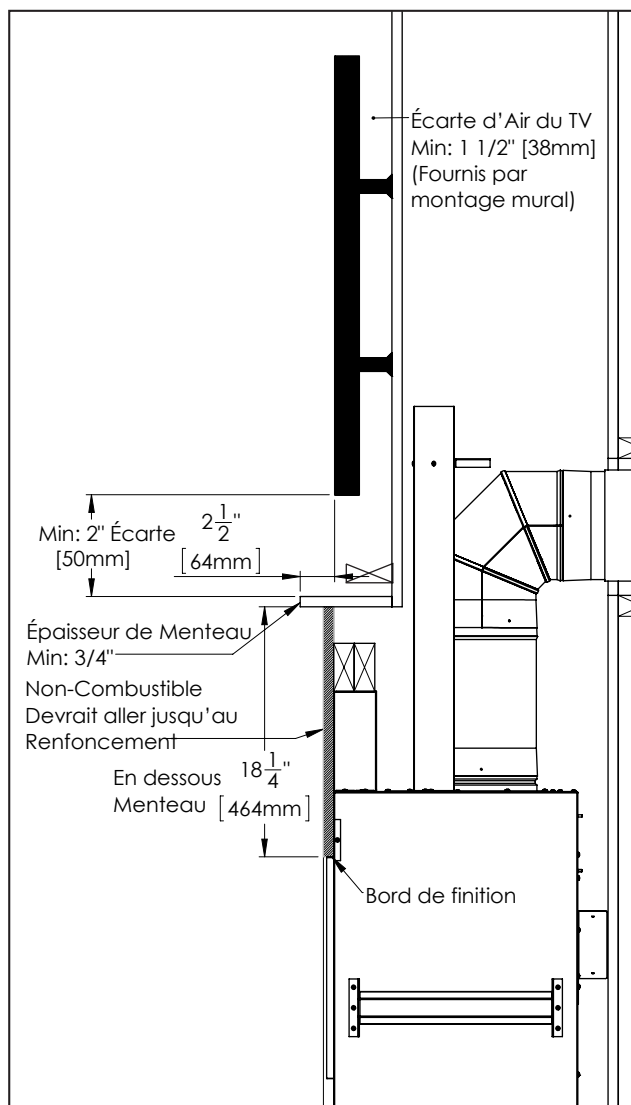
Figure 38. Dégagement minimum d'Installation de TV avec renforcement
