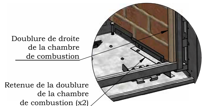
Coin inférieur droit de la chambre de combustion
