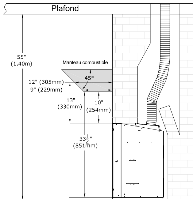
Dégagements du manteau combustible (ci-dessus) Dégagements du manteau incombustible (ci-dessous)
