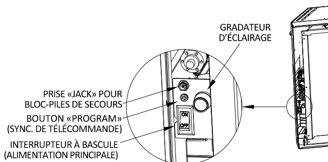
Figure 11.1 - Panneau du module de contrôle
