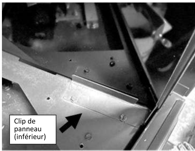
Figure 9.7 - Clip (inférieur) de panneau en verre noir
