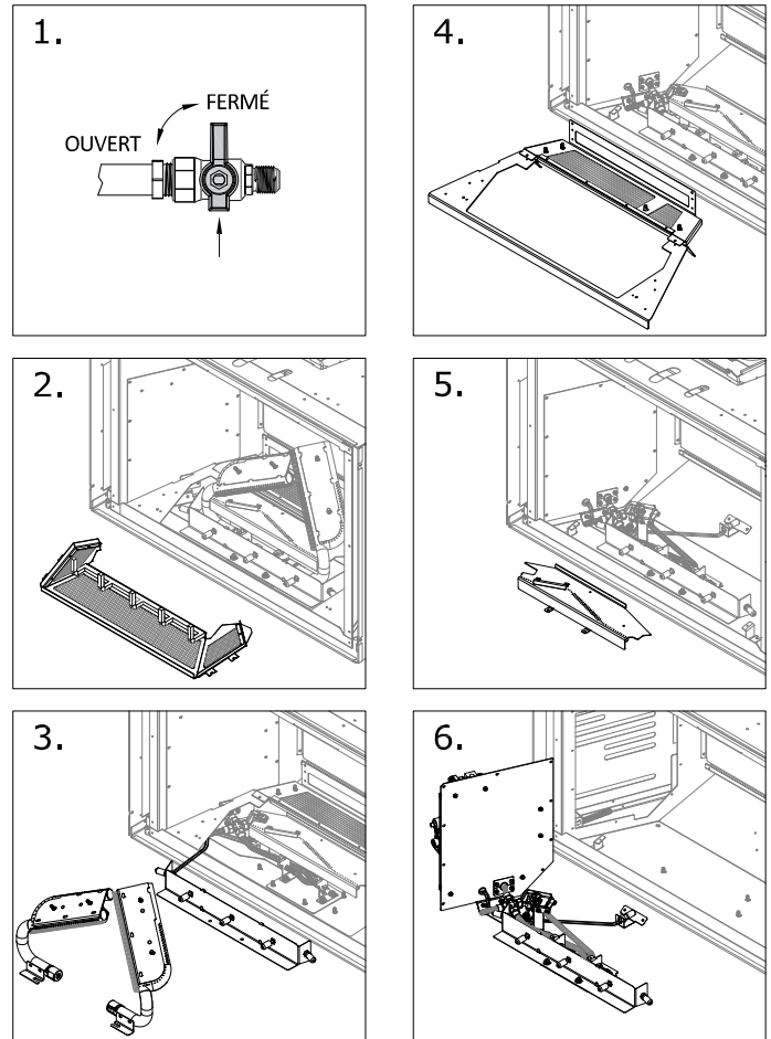
Figure 9.8 - Retrait du panneau de contrôle
