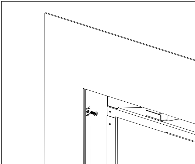
Figure 9.9 - Brides et écrous de fixation alignés
