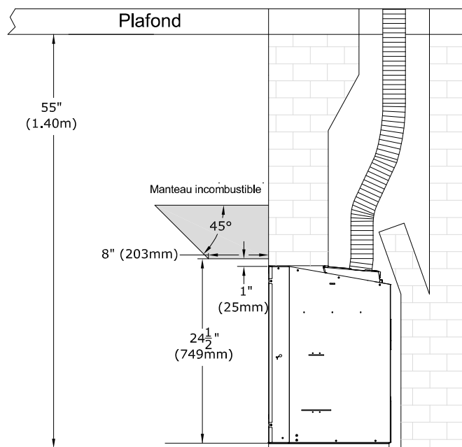
Figure 8.4 - Exigences d'installation du manteau
