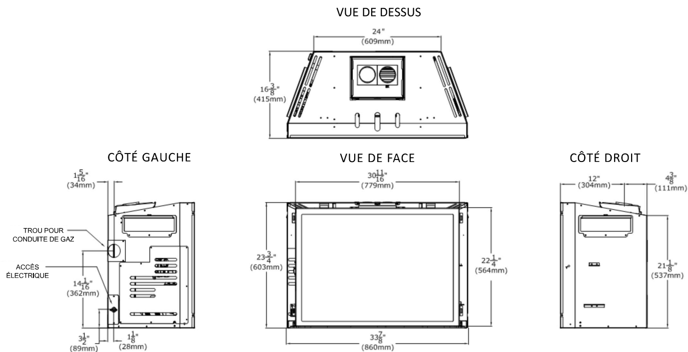
Figure 2.1 - Dimensions de l'appareil
