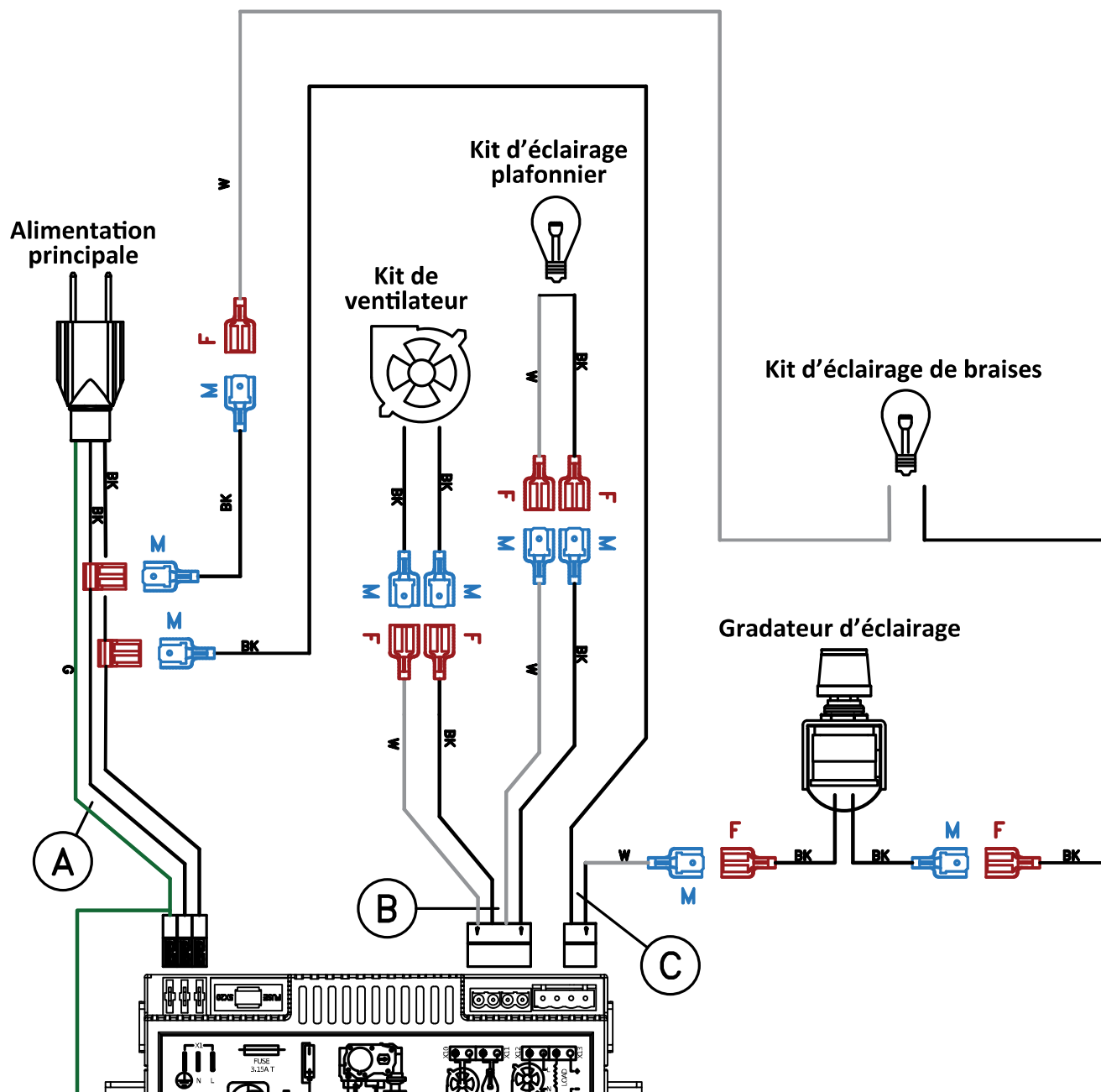
Figure 10.2 - Schéma électrique - Vue agrandie (1)
