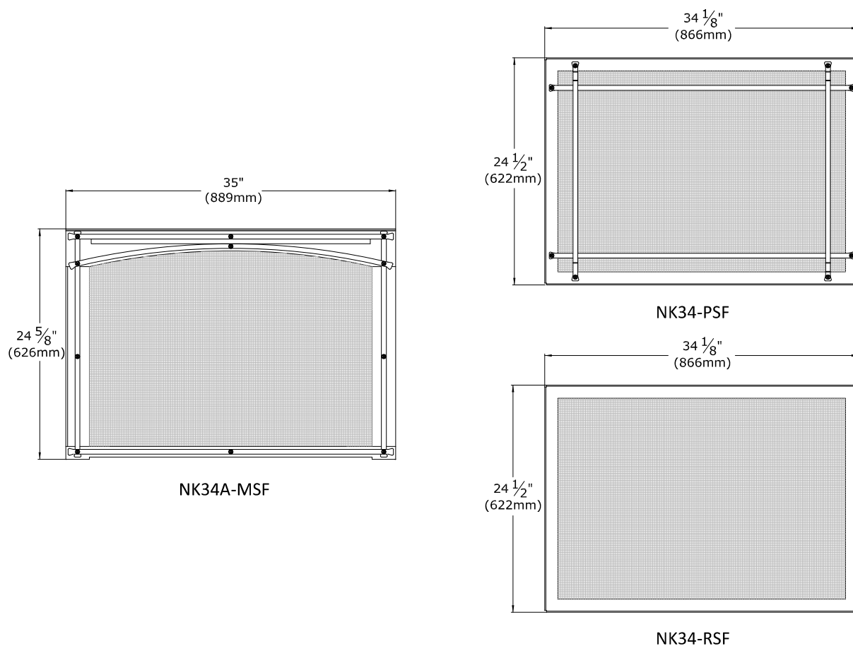
Figure 2.3 - Dimensions des écrans pare-étincelles
