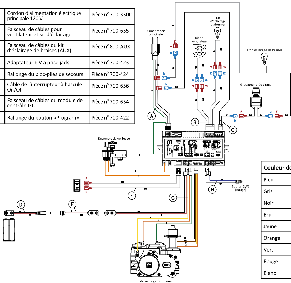
Figure 10.1 - Schéma de câblage
