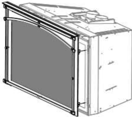
Figure 9.10 - Installation de l'écran pare-étincelles
