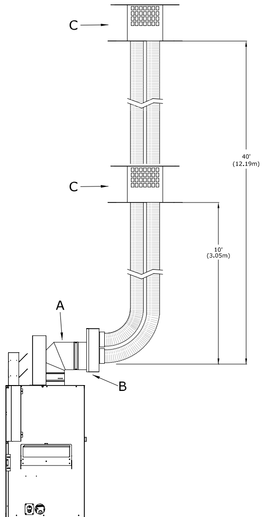
Figure 8.8 - Conversion de conduit coaxial à colinéaire
