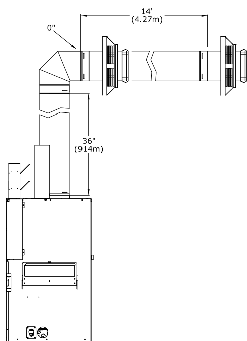
Figure 8.5 - Conduit 4 po x 6-5/8 po à terminaison horizontale
