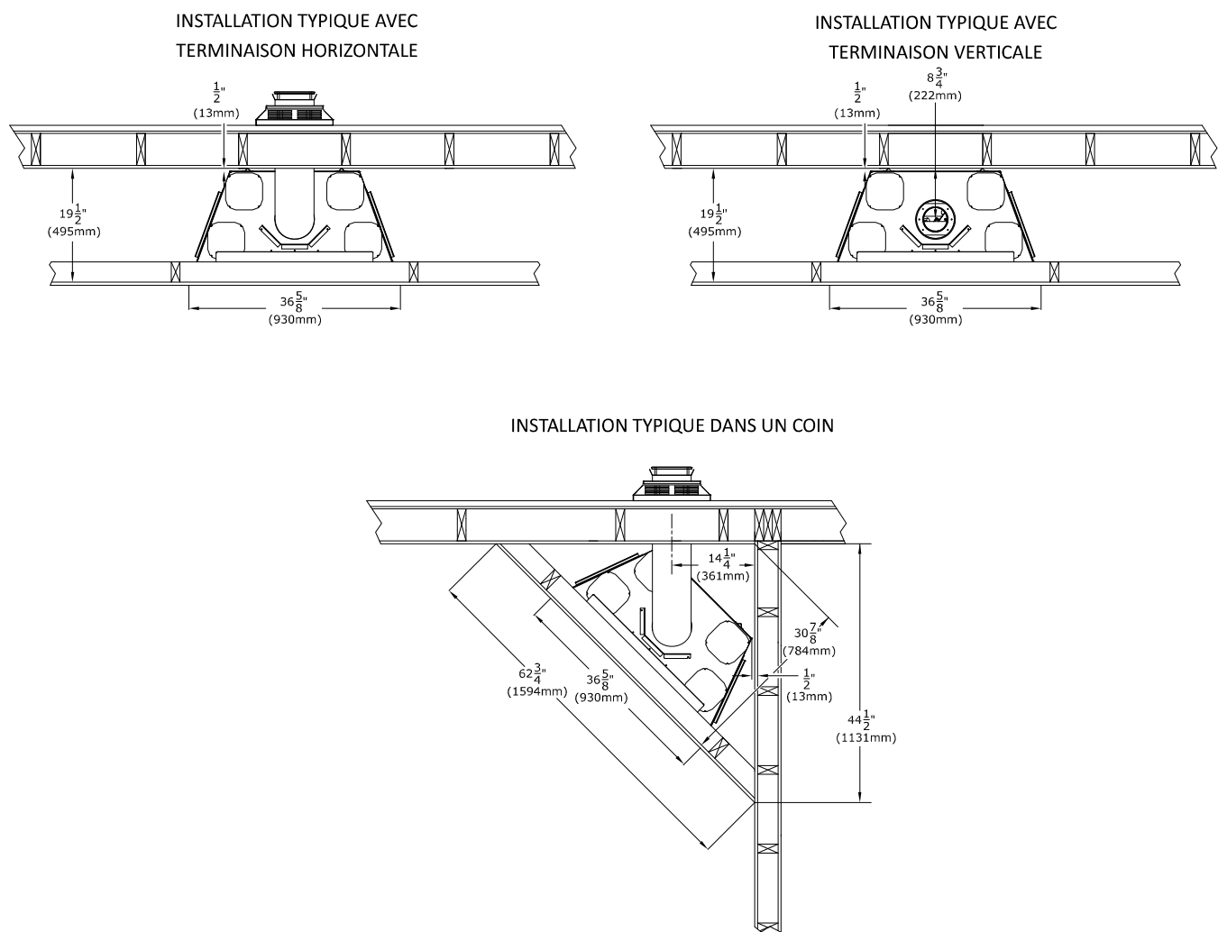
Figure 3.3 - Installations typiques de l'appareil
