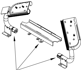
Venturis des brûleurs
