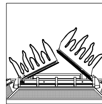
Flammes orange foncé - Réglage de venturis requis
