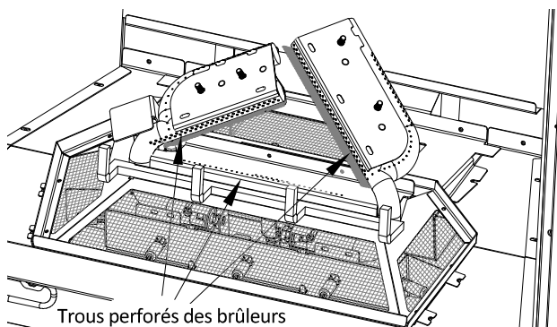
Figure 14.1 - Système de brûleurs
