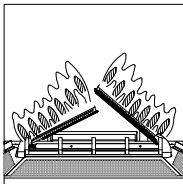
Flammes sautillantes («ghosting») (Venturis trop fermés. Ouvrir légèrement les venturis.) OU (Pression de gaz trop élevée - vérifier la pression avec le manomètre)
