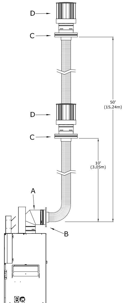
Figure 8.7 - Conversion de cheminée (Classe A/maçonnerie)
