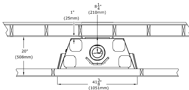
INSTALLATION TYPIQUE AVEC TERMINAISON VERTICALE
