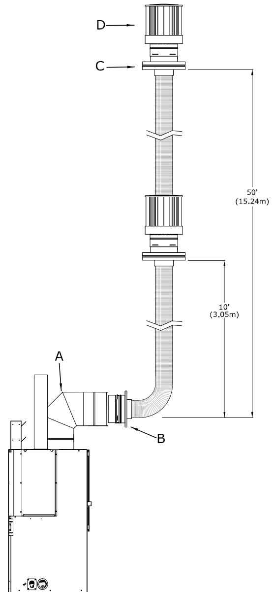
Figure 8.9 - Conversion de cheminée (Classe A/maçonnerie)
