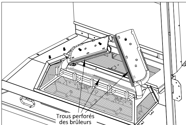
Figure 14.1 - Système de brûleurs
