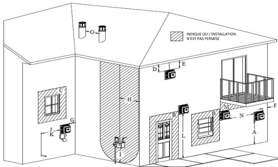
Figure 7.3 - Dégagements des terminaisons d'évacuation
