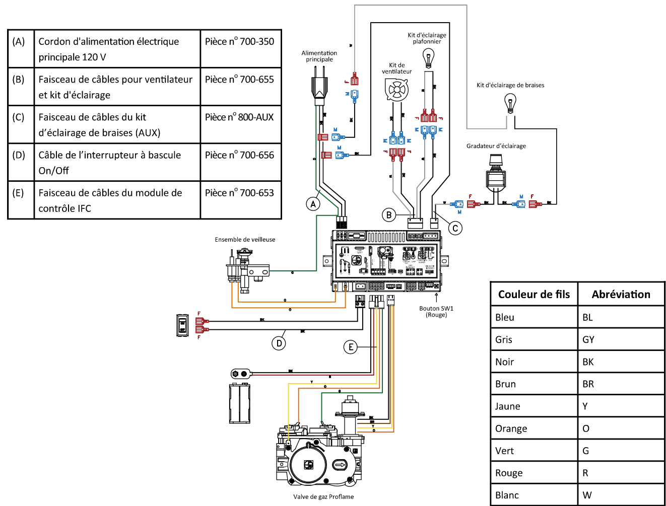
Figure 10.1 - Schéma électrique
