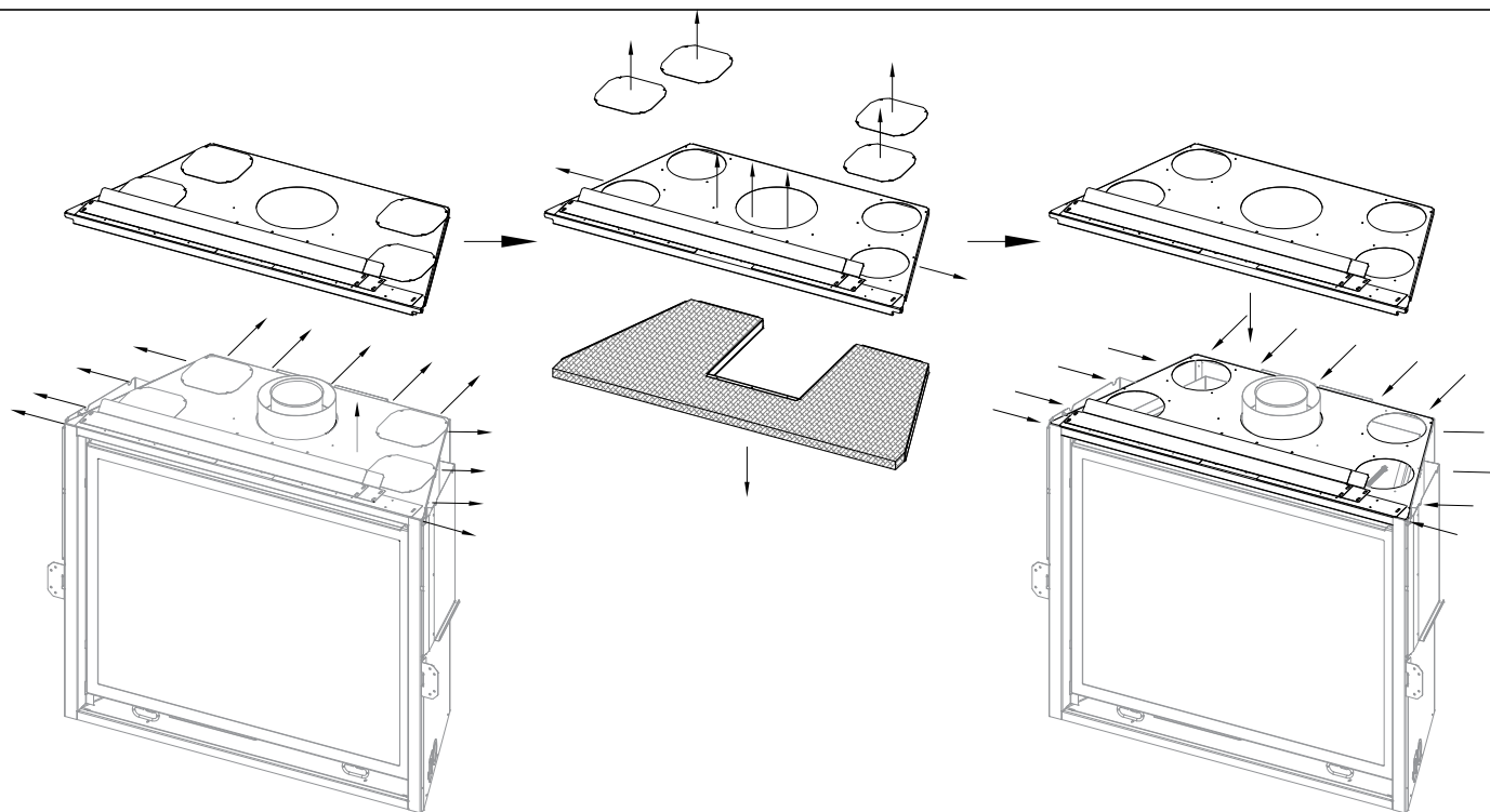
Figure 4.1 - Retrait de la plaque du dessus et de l'isolant
