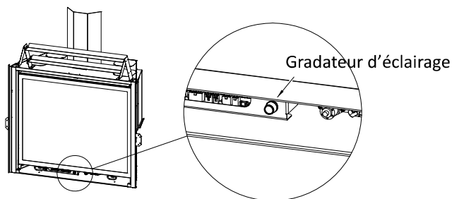
Figure 11.15 - Gradateur d'éclairage du lit de braises
