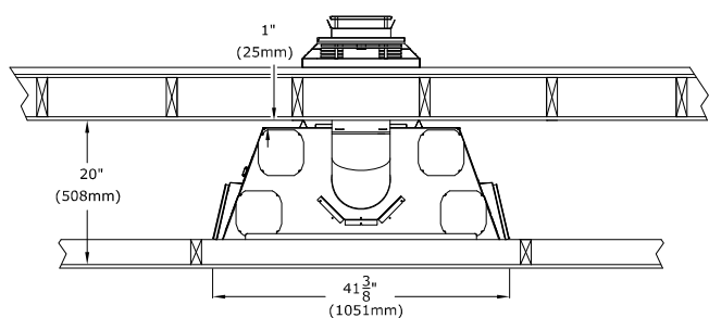
INSTALLATION TYPIQUE AVEC TERMINAISON HORIZONTALE
