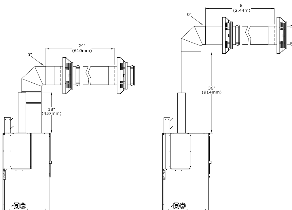
Figure 8.5 - Conduit 5 po x 8 po à terminaison horizontale
