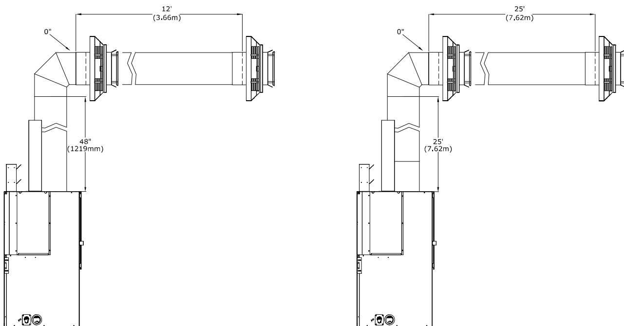
Figure 8.6 - Conduit 5 po x 8 po à terminaison horizontale
