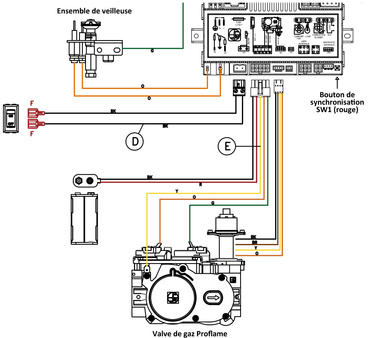
Figure 10.3 - Schéma électrique - Vue agrandie (2)
