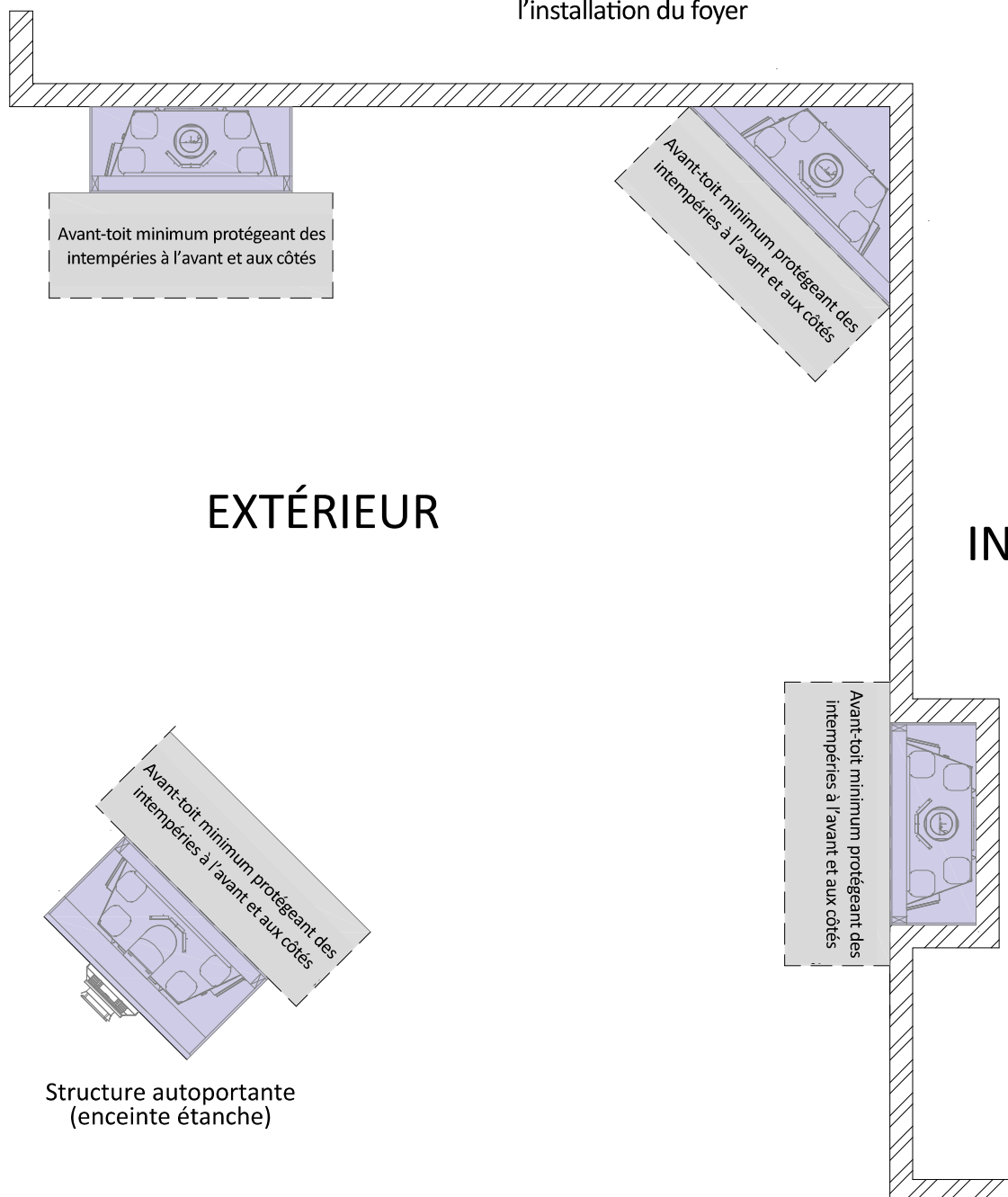
Figure 3.8 - Installation du foyer extérieur couvert
