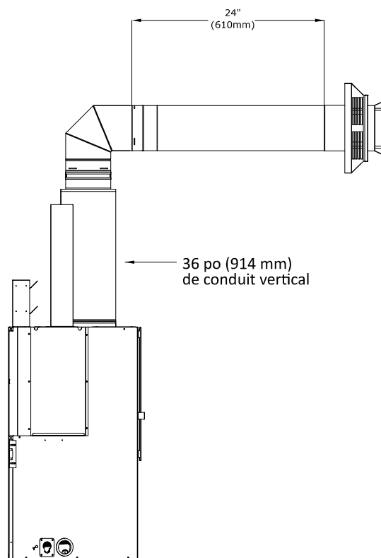
Figure 8.7 - Conduit 4 po x 6-5/8 po à terminaison horizontale
