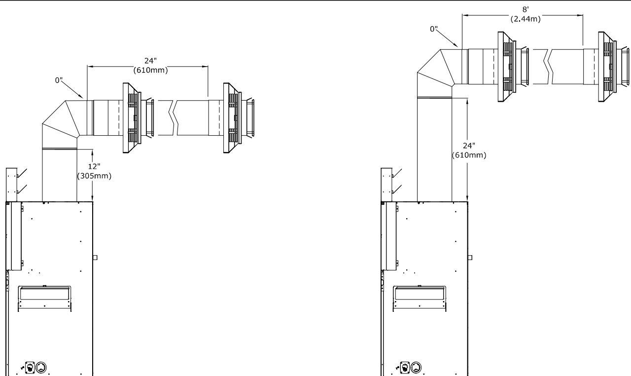
Figure 8.4 - Conduit 4 po x 6-5/8 po à terminaison horizontale
