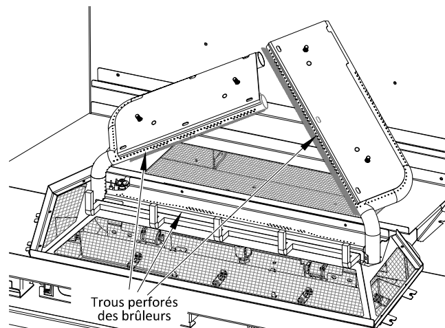
Figure 14.1 - Système de brûleurs
