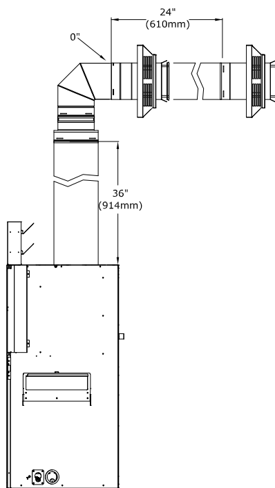
Figure 8.6 - Installation dans un sous-sol : Conduit 4 po x 6-5/8 po à terminaison horizontale
