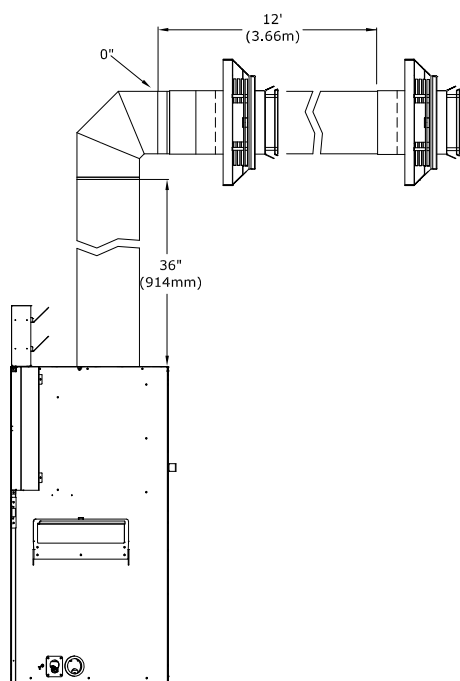
Figure 8.5 - Conduit 5 po x 8 po à terminaison horizontale
