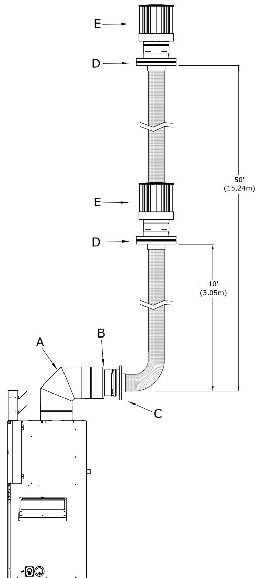
Figure 8.8 - Conversion de cheminée (Classe A/maçonnerie)
