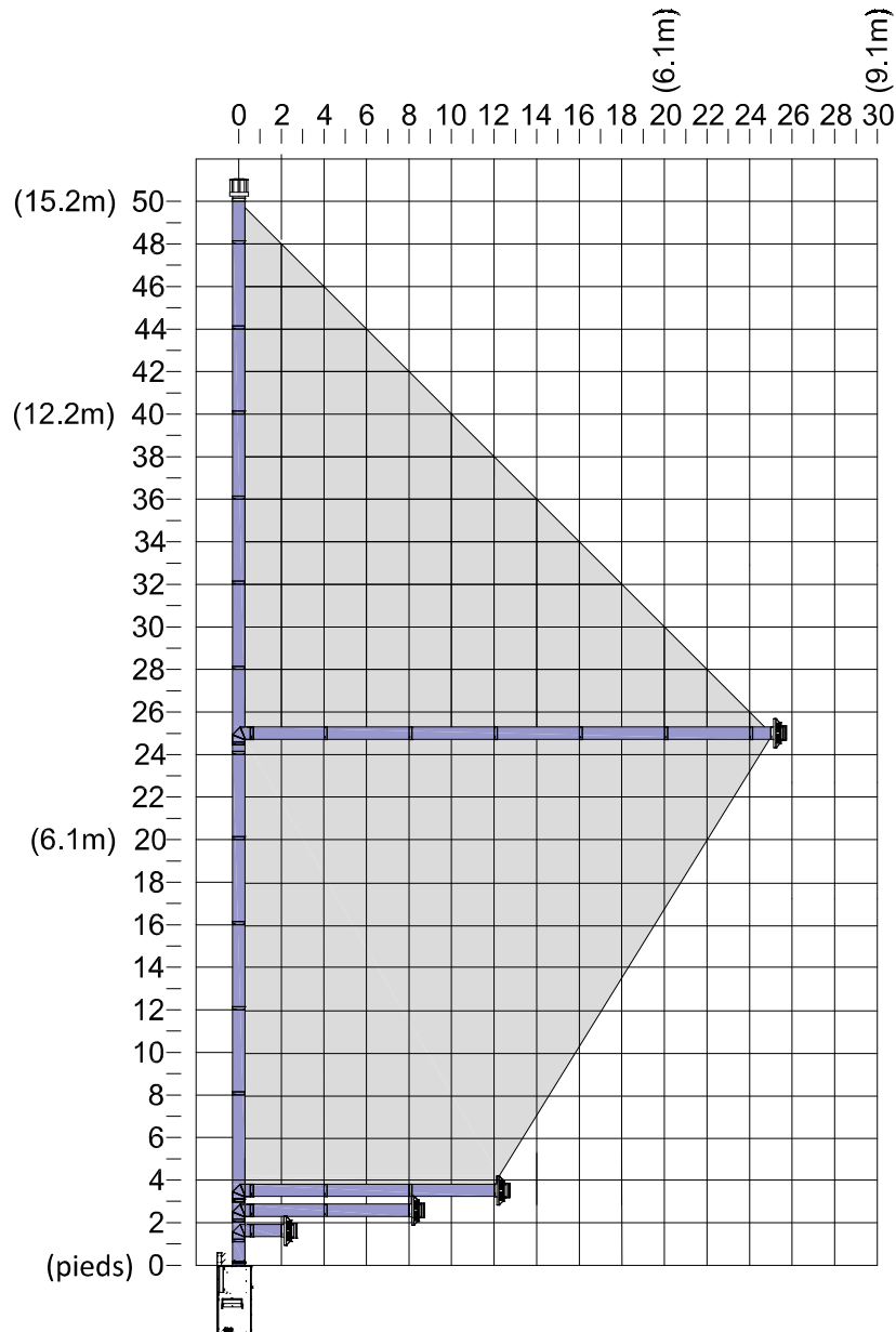
Figure 8.7 - Diagramme d'évacuation pour conduits 5 po x 8 po combinés (V/H)
