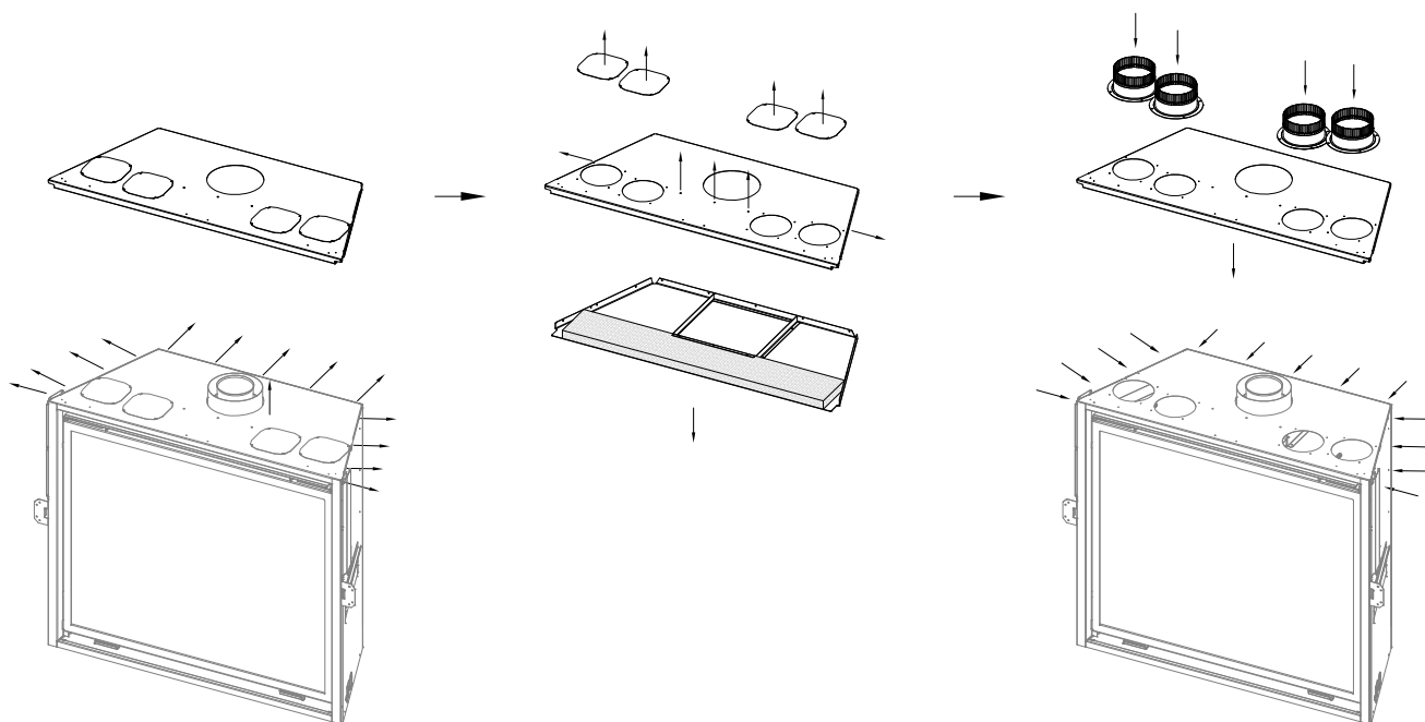
Figure 4.1 - Retrait de la plaque du dessus et de l'isolant
