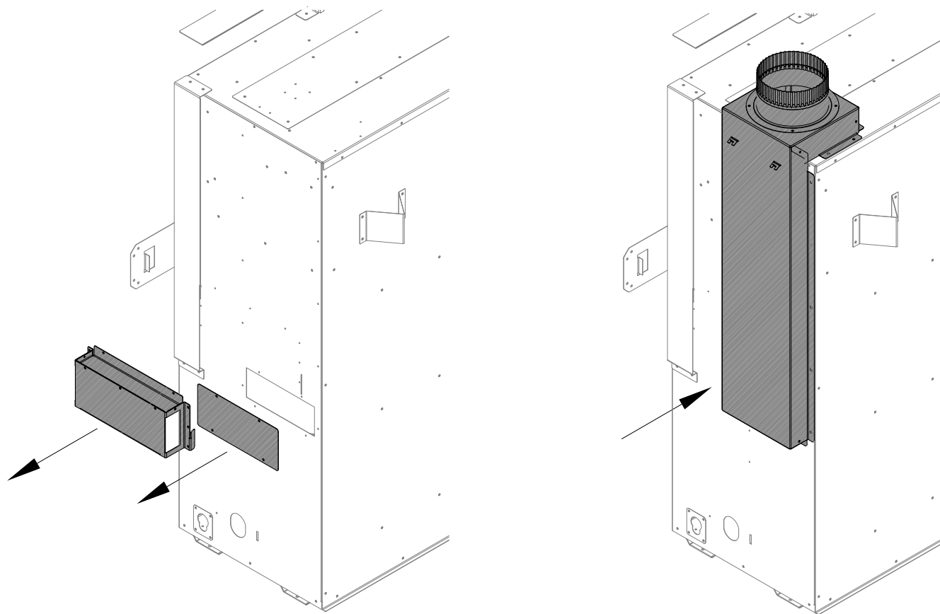
Figure 4.4 - Installation de la chute d'air du kit HTK
