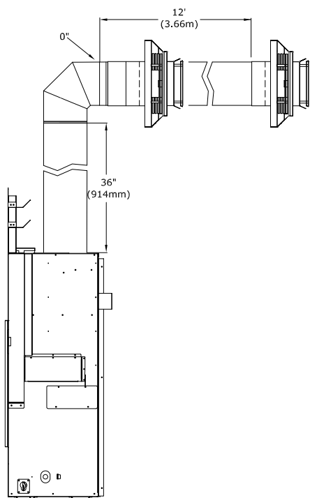
Figure 8.5 - Conduit 5 po x 8 po à terminaison horizontale
