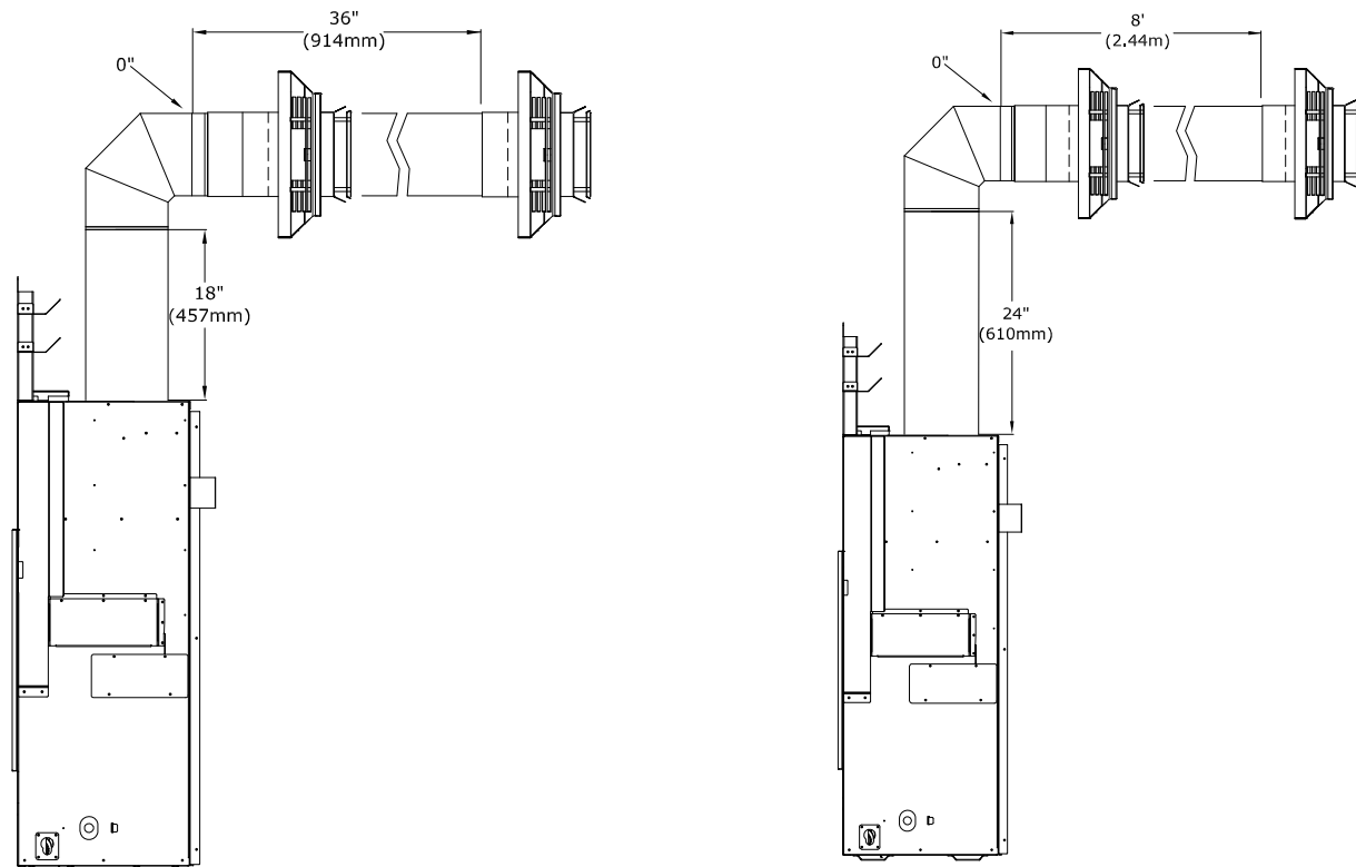
Figure 8.4 - Conduit 5 po x 8 po à terminaison horizontale
