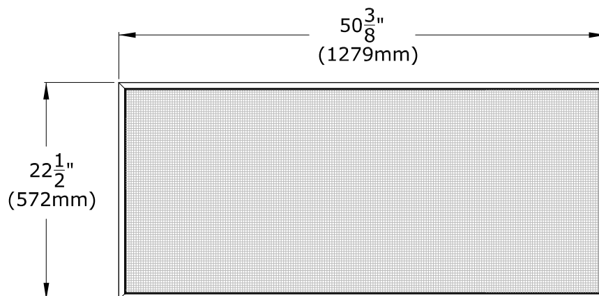
Écran pare-étincelles NK48TL-ES
