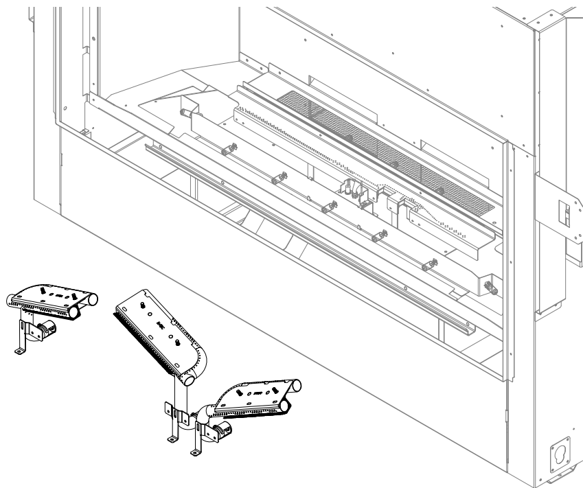
Figure 9.4 - Retrait des brûleurs gauche, central et droit
