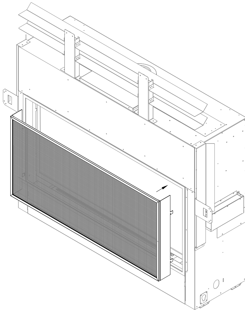
Figure 5.8 - Installation de l'écran pare-étincelles
