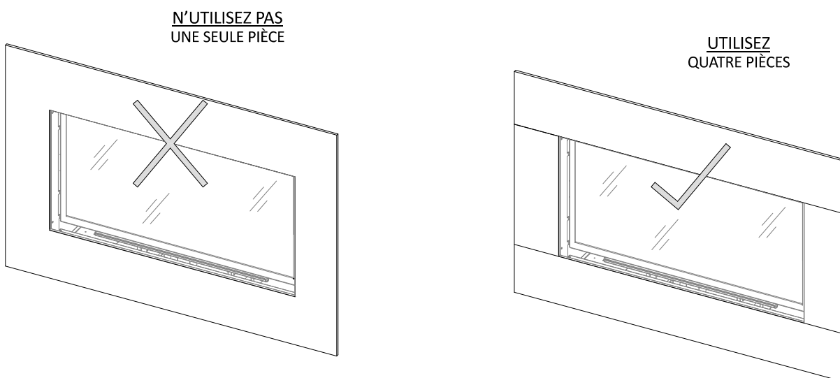
Figure 5.1 - Exemple d'installation du marbre
