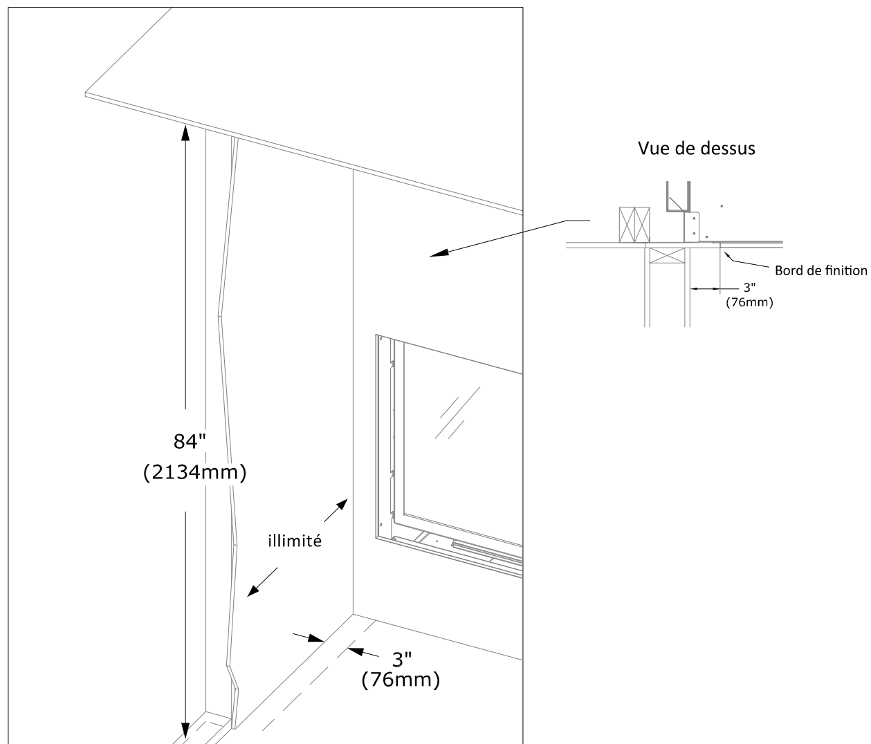
Figure 5.5 - Projection d'un mur latéral combustible
