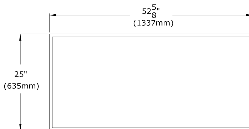
Contour rectangulaire (en option) NK48TL-RS
