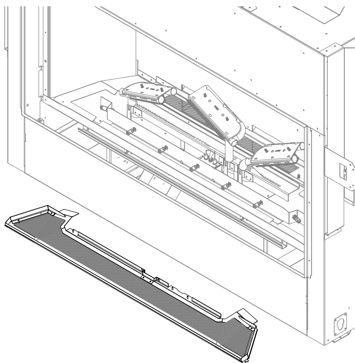
Figure 9.3 - Retrait du plateau à braises (à l'avant)
