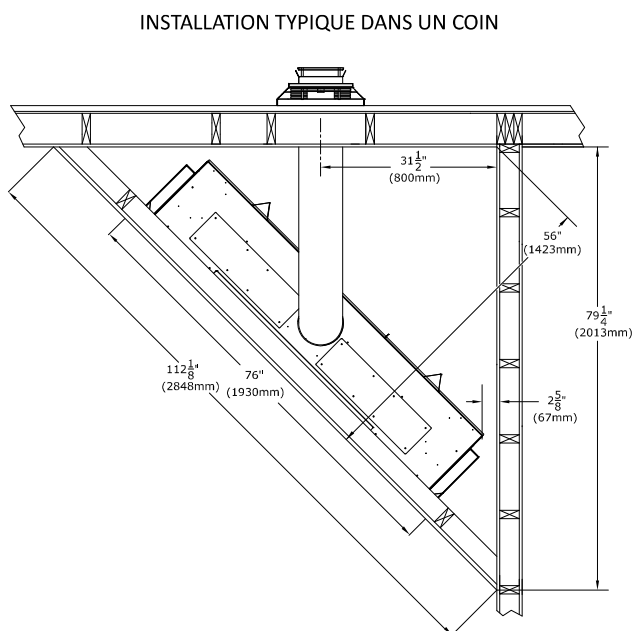
Figure 3.3 - Installations typiques de l'appareil
