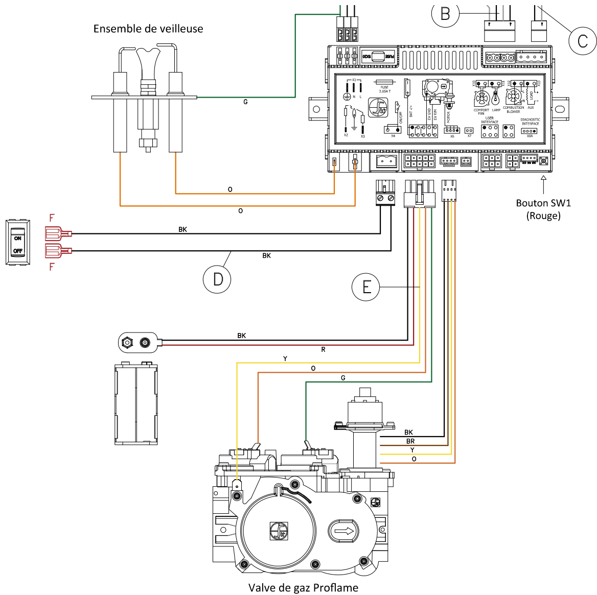
Figure 10.3 - Schéma électrique (Vue agrandie 2)
