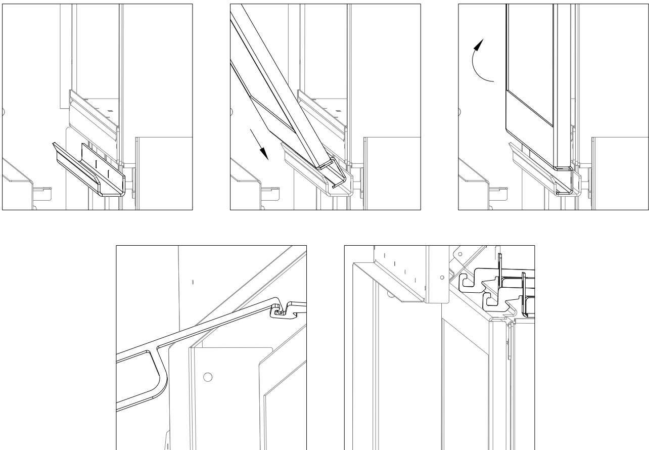
Figure 9.1 - Installation du cadre vitré
