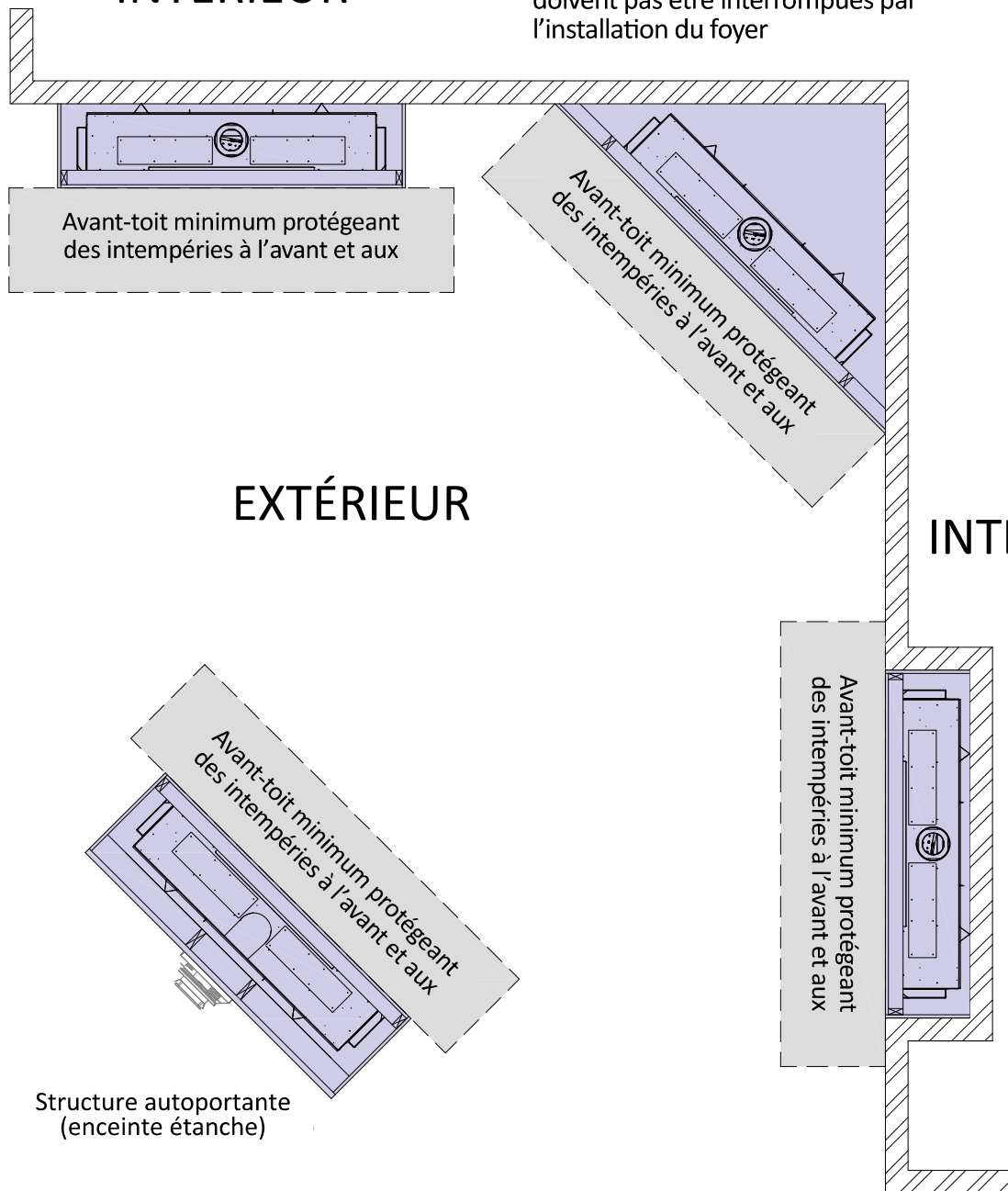
Figure 3.9 - Installation du foyer extérieur couvert
