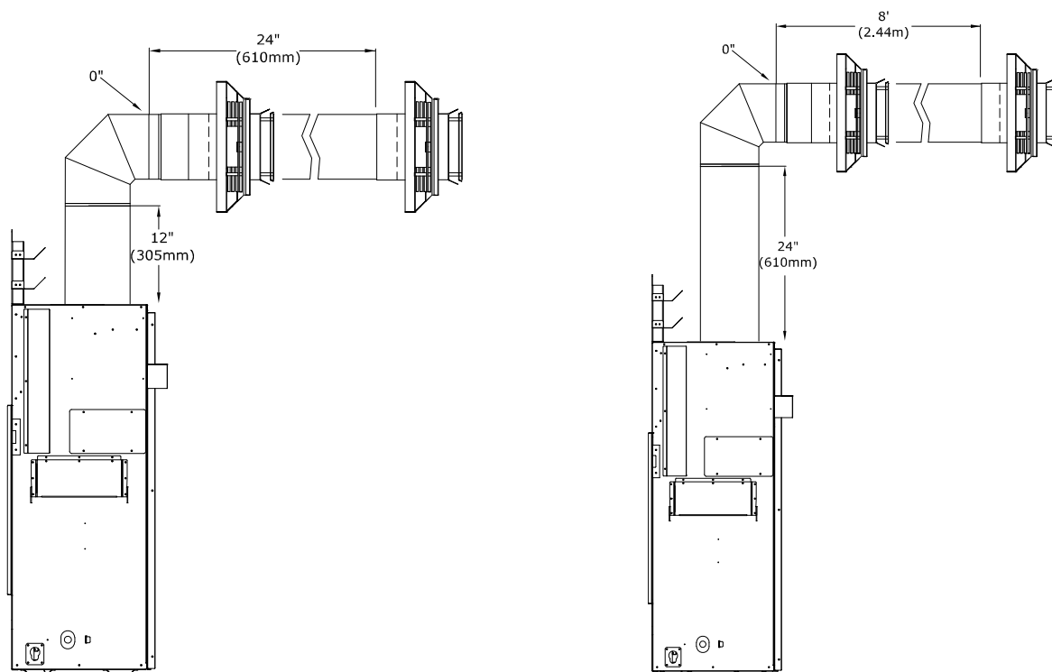
Figure 8.4 - Conduit 4 po x 6-5/8 po à terminaison horizontale
