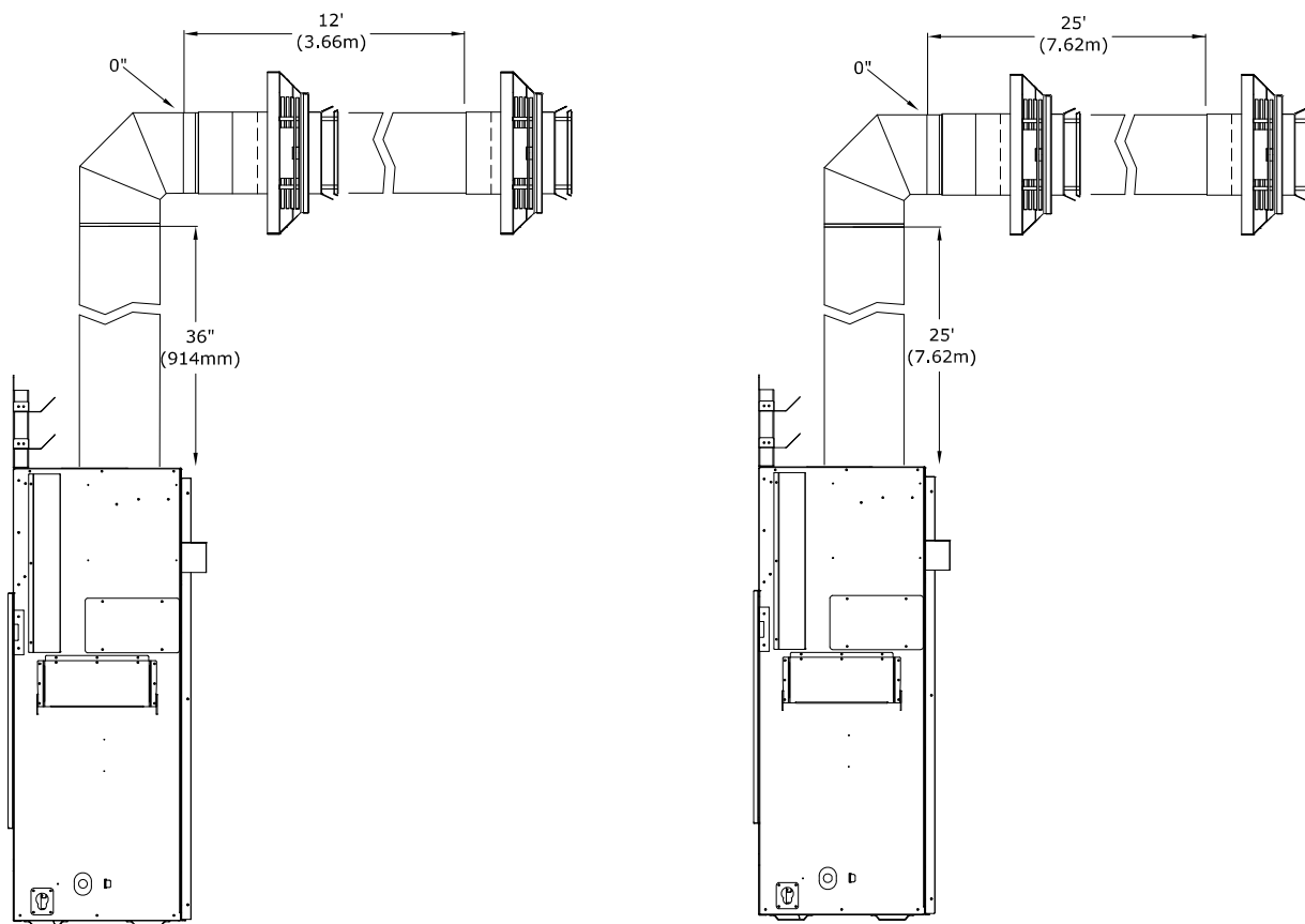
Figure 8.5 - Conduit 5 po x 8 po à terminaison horizontale
