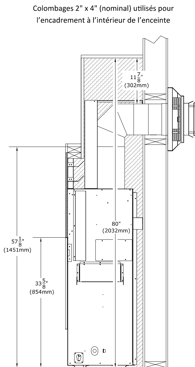
Figure 3.5 - Dégagements du conduit d'évacuation horizontal
