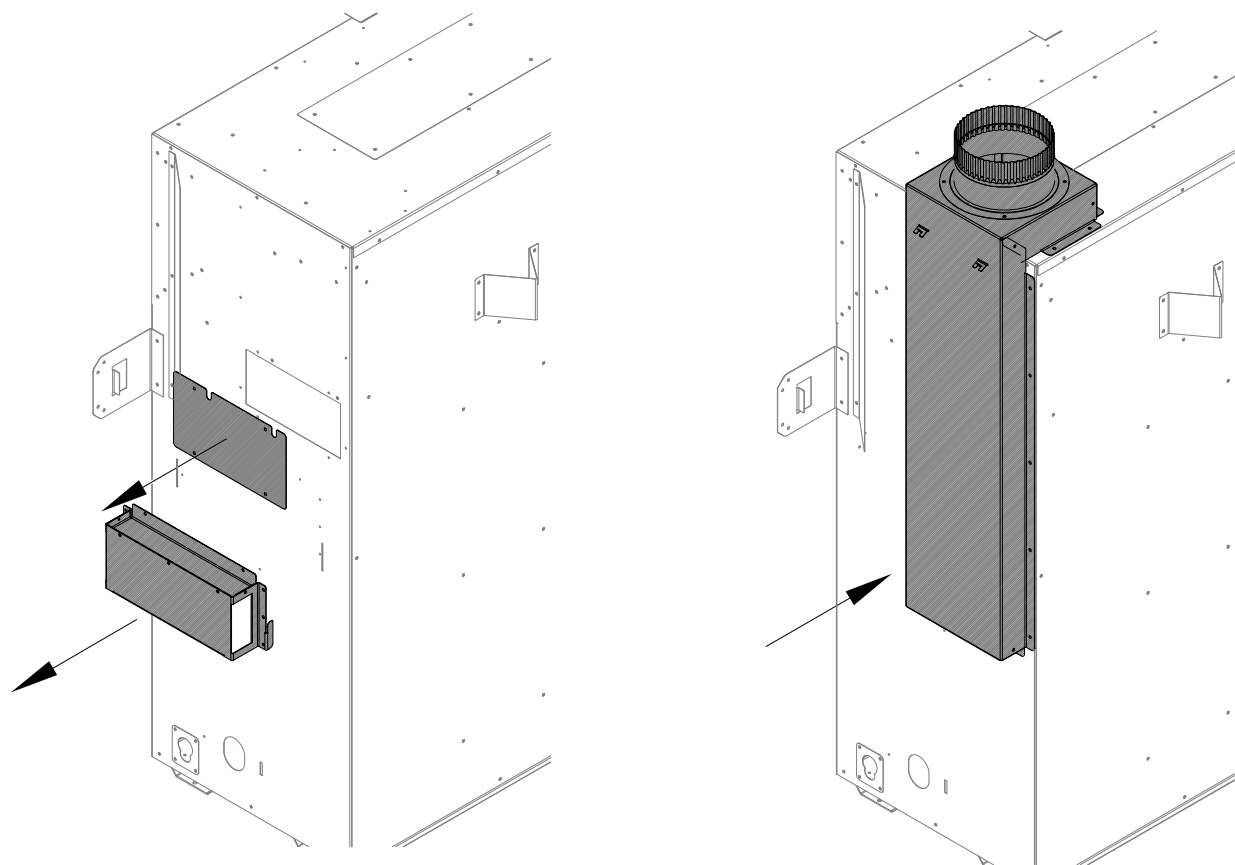
Figure 4.4 - Installation de la chute d'air du kit HTK
