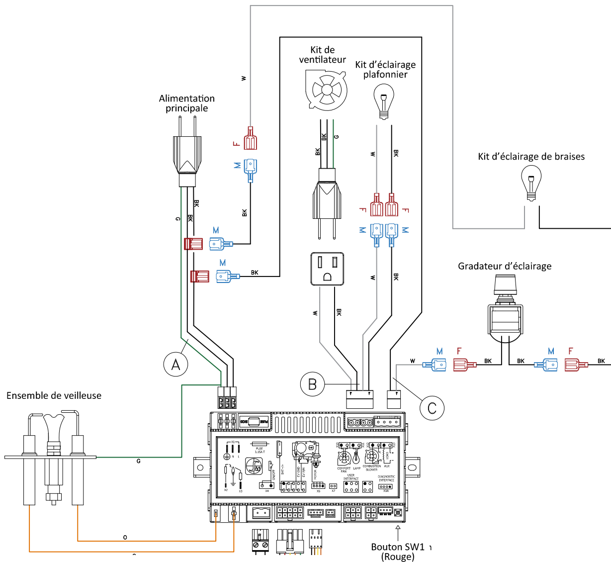
Figure 10.2 - Schéma électrique (Vue agrandie 1)
