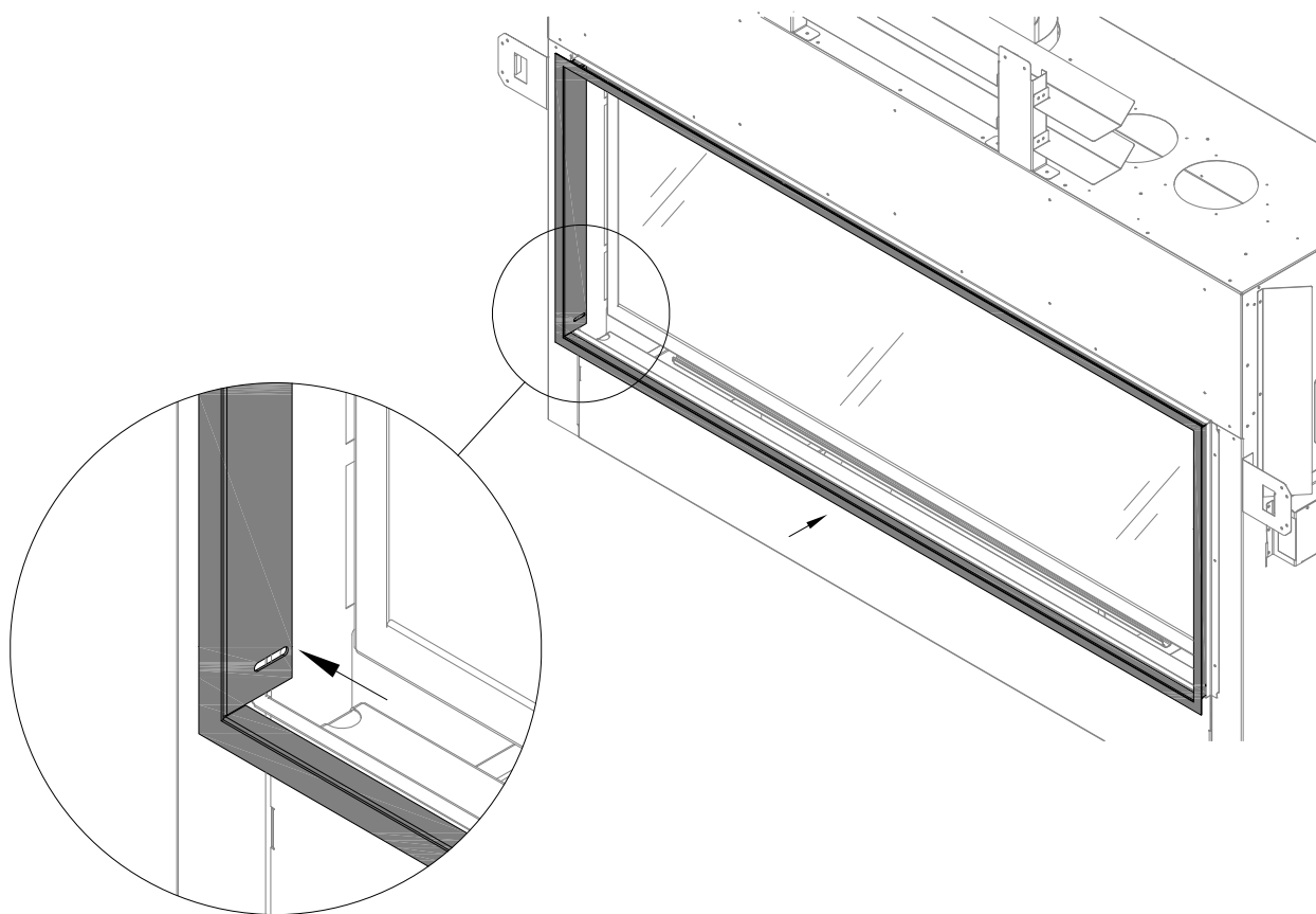
Figure 5.7 - Installation du contour rectangulaire
